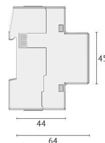
Abmessungen (mm):
